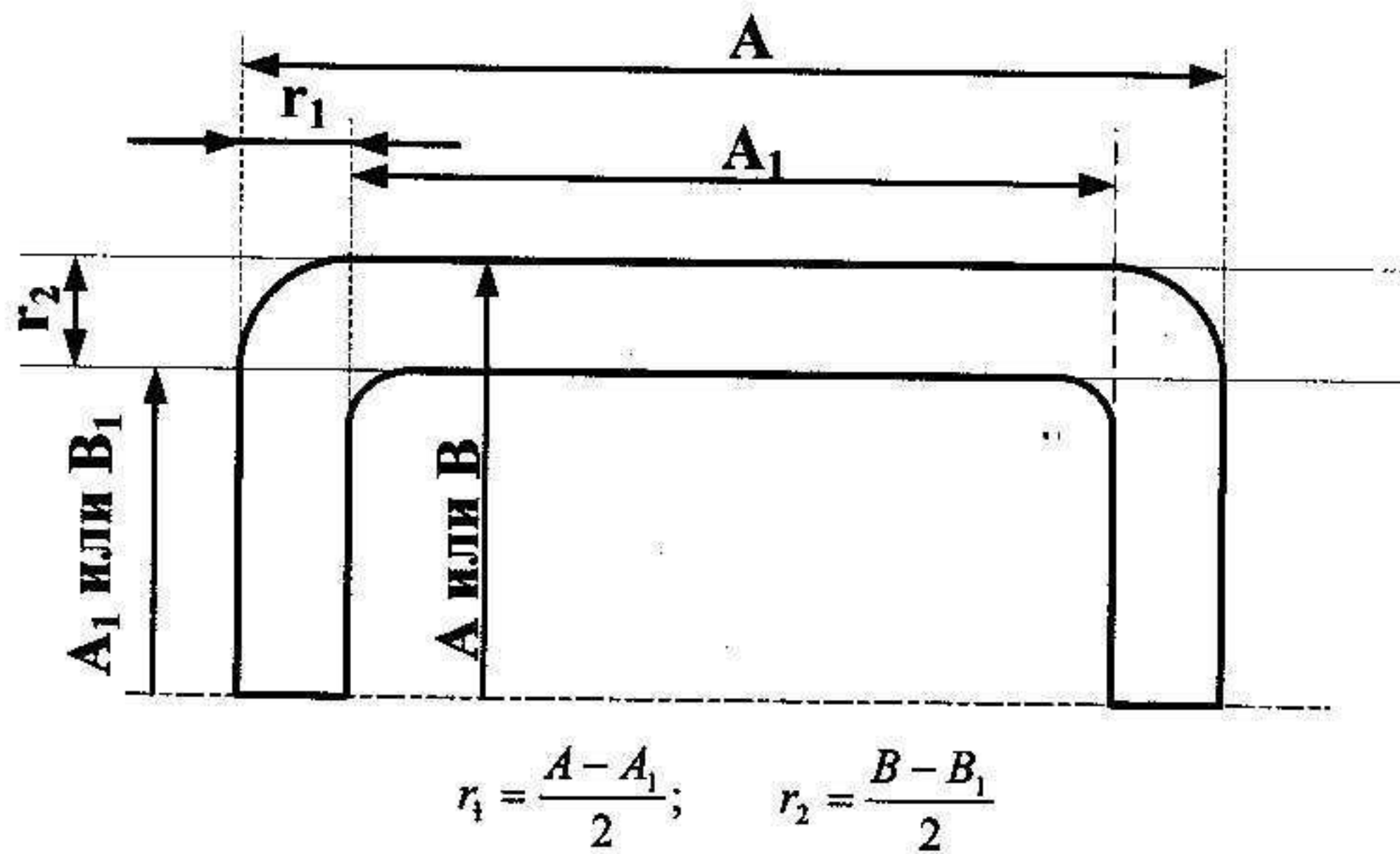
Рис. 7 Внешнее скругление угла (зона кромки)
