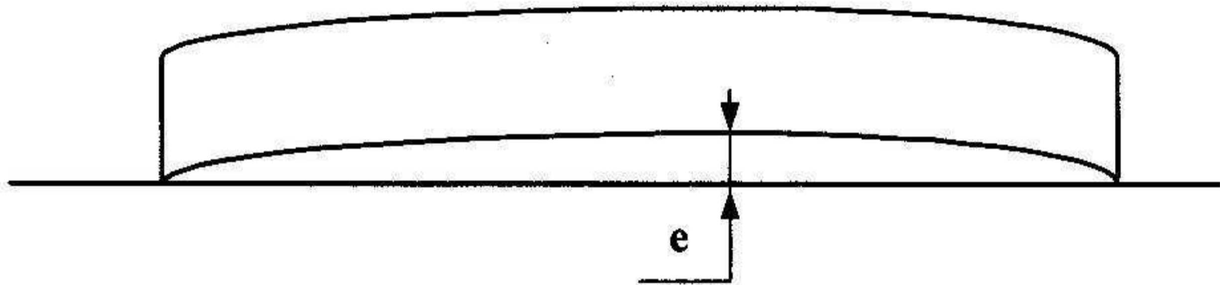
Рис. 9 Отклонение от прямолинейности (кривизна)
